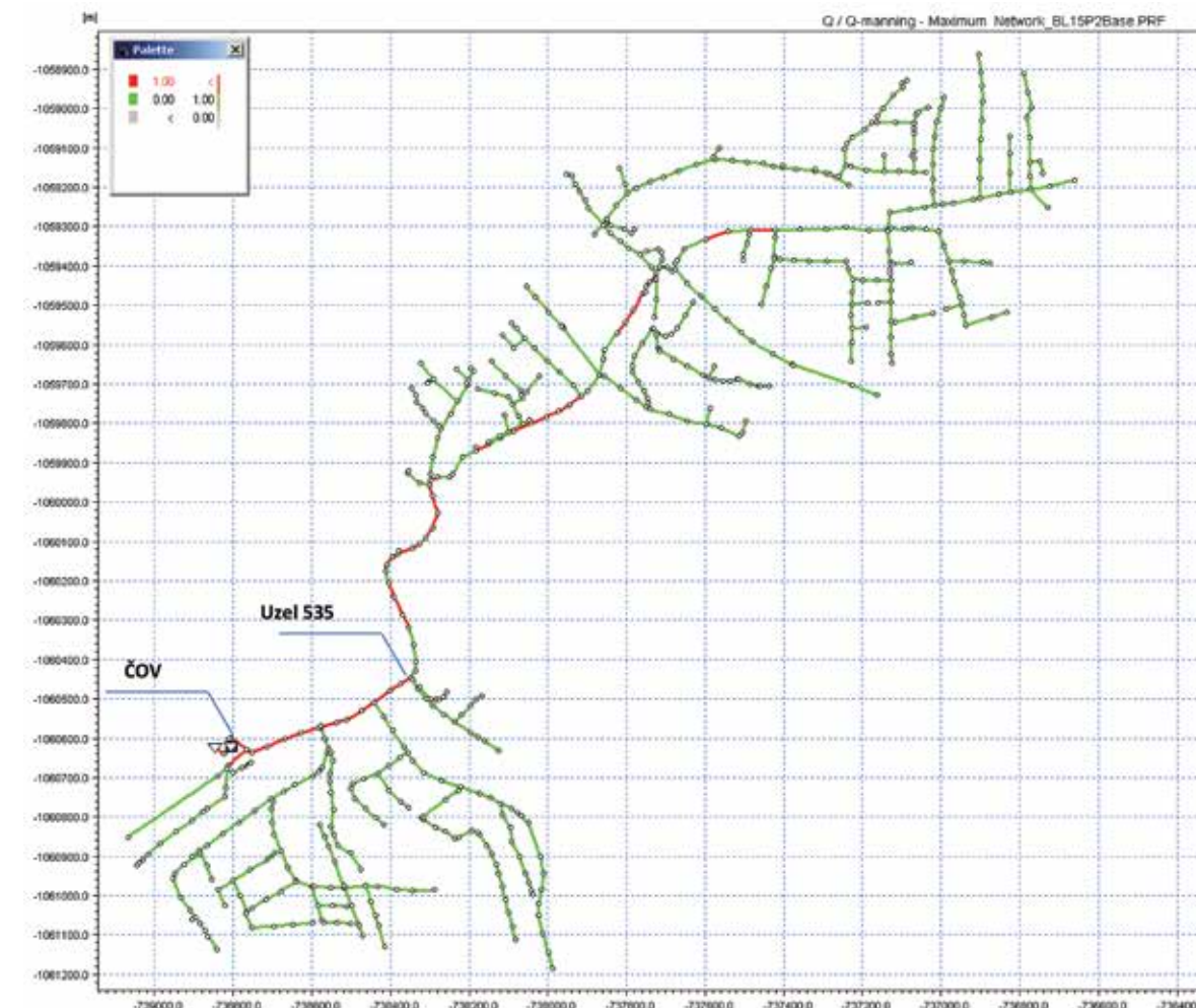
Výsledné hydraulické posouzení poměru Q_{max}/Q_{kap}
