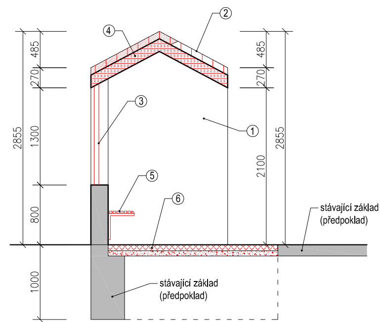
Řez A-A
