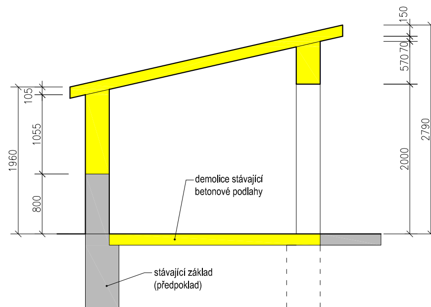
Řez A-A
