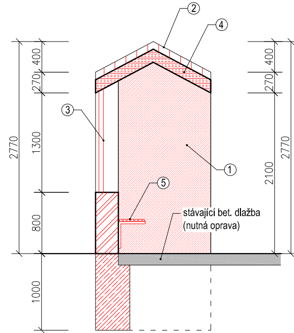
Řez A-A
