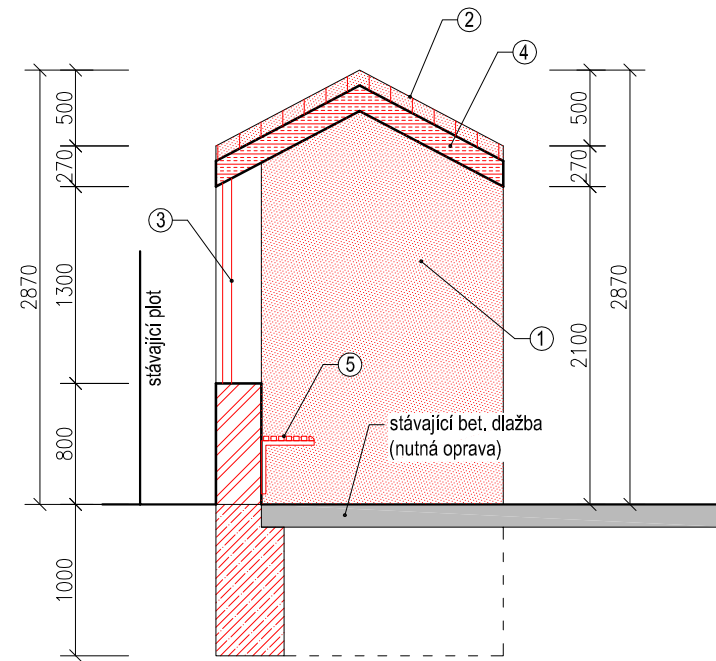
Řez A-A
