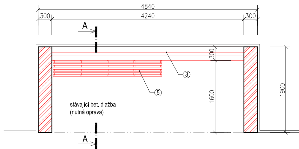
Půdorys
